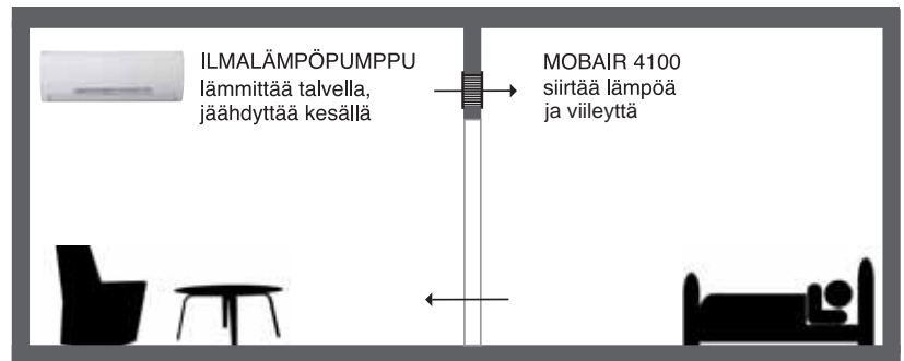
MOBAIR 4100 toimintaperiaate
