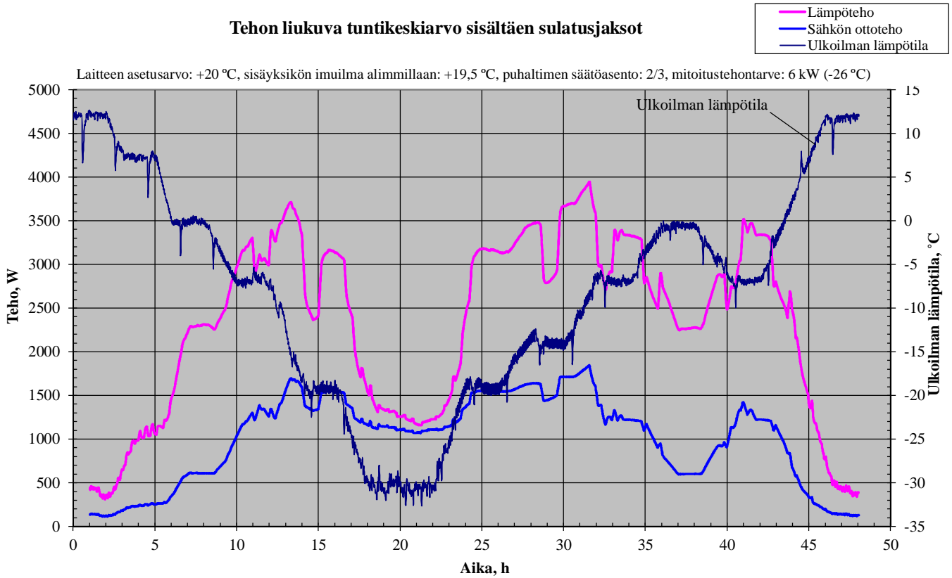
Hetkellinen teho
